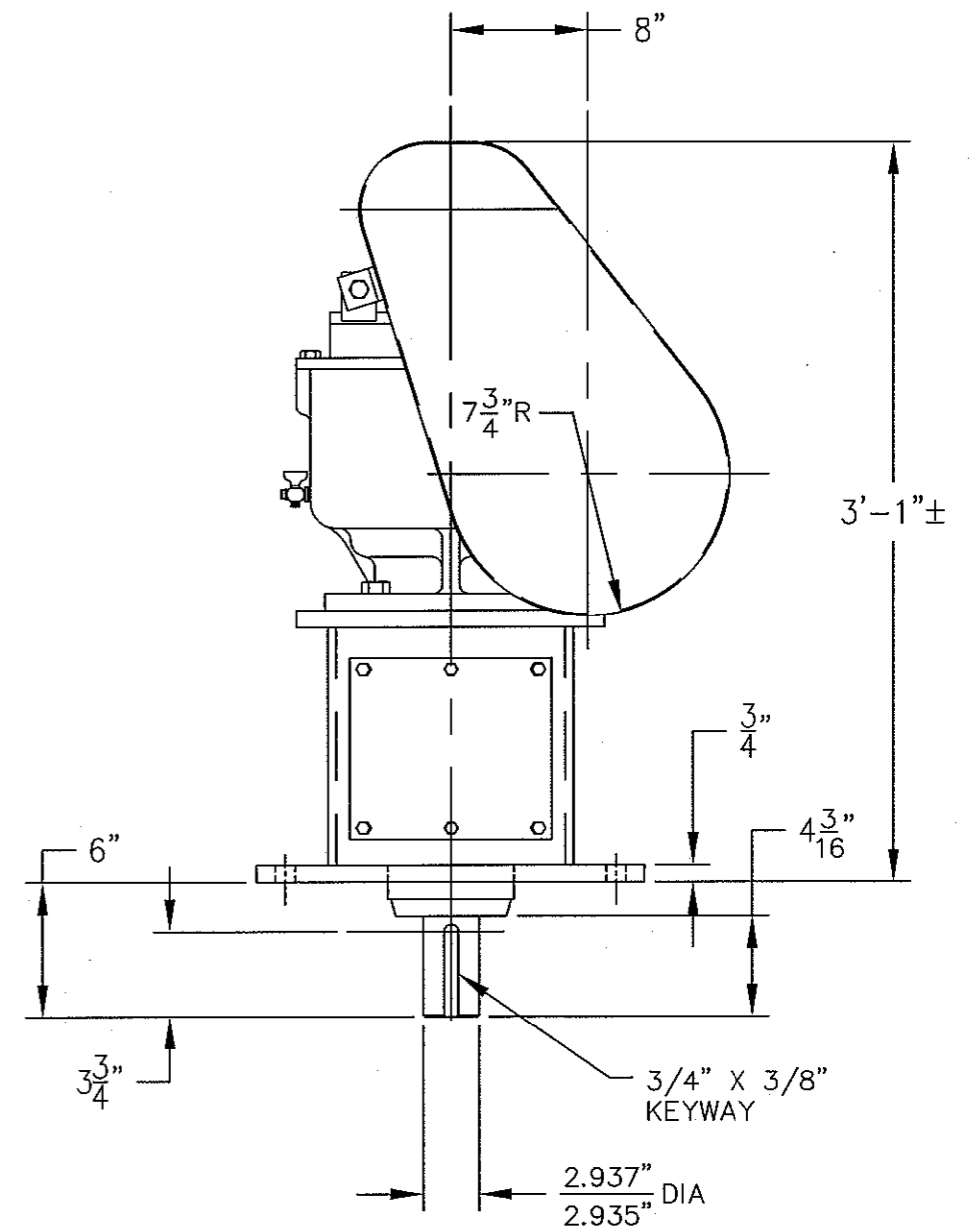
ELEVATION
